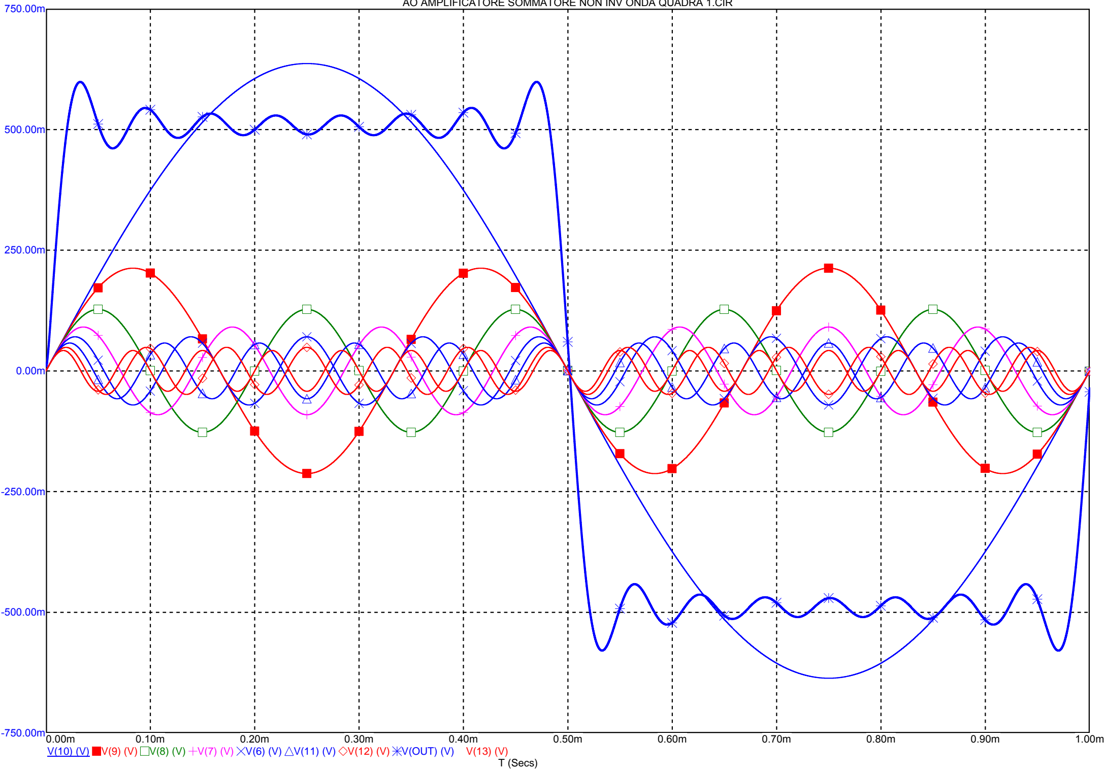
Micro-Cap 9 Evaluation Version AO AMPLIFICATORE SOMMATORE NON INV ONDA QUADRA 1.CIR
